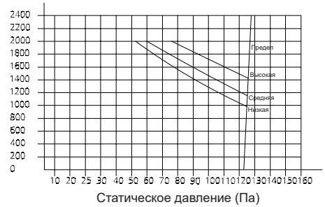
Объем воздуха, м³/ч (без фильтра) SP4
