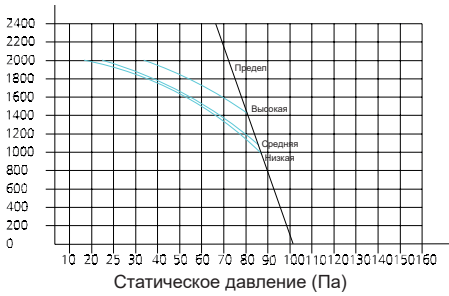
Объем воздуха, м³/ч (без фильтра) SP3
