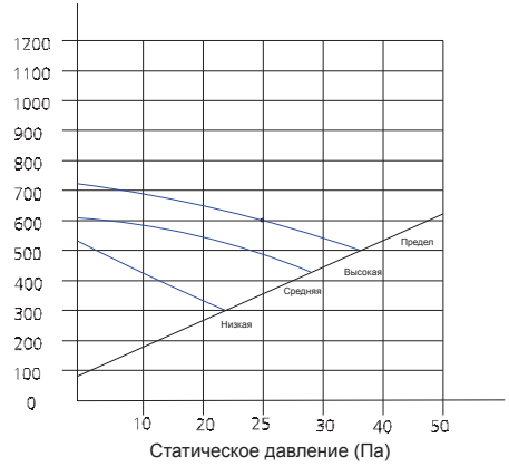
Объем воздуха, м³/ч SP4
