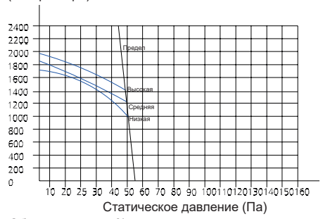
Объем воздуха, м³/ч (без фильтра) SP4
