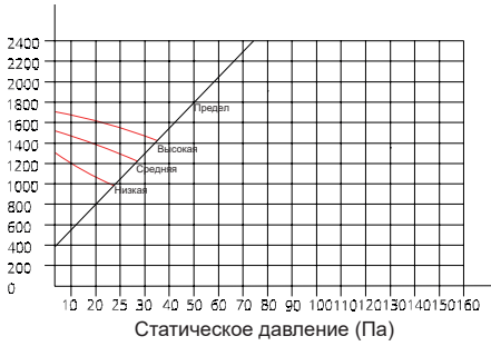
Объем воздуха, м³/ч (без фильтра) SP3
